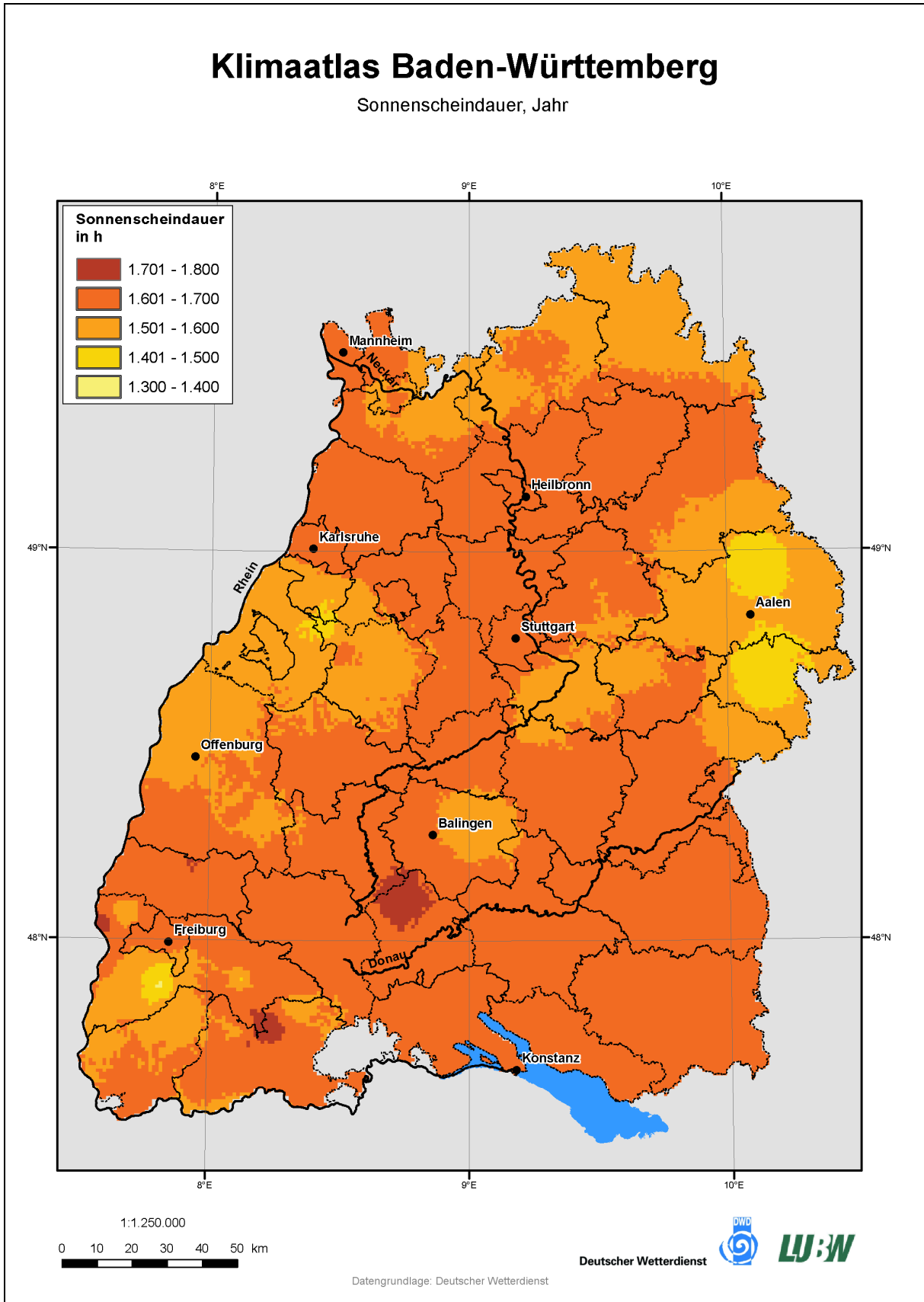
Karte 9: Jährliche Sonnenscheindauer in Baden-Württemberg (LUBW, 2006).
