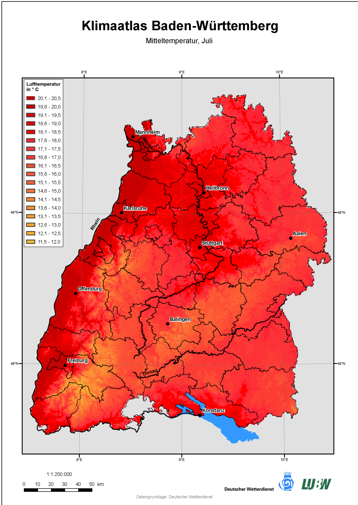
Karte 3: Mittelwert der Lufttemperaturen im Juli in Baden-Württemberg (LUBW, 2006).
