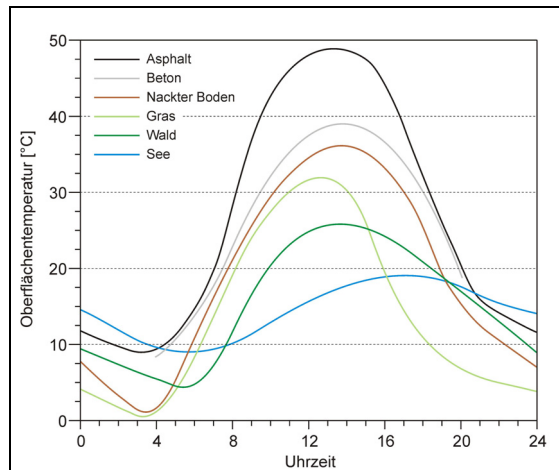
Abbildung 3: Typischer Tagesgang der Oberflächentemperaturen verschiedener Oberflächen (verändert nach Häckel, 1999, S.226).
