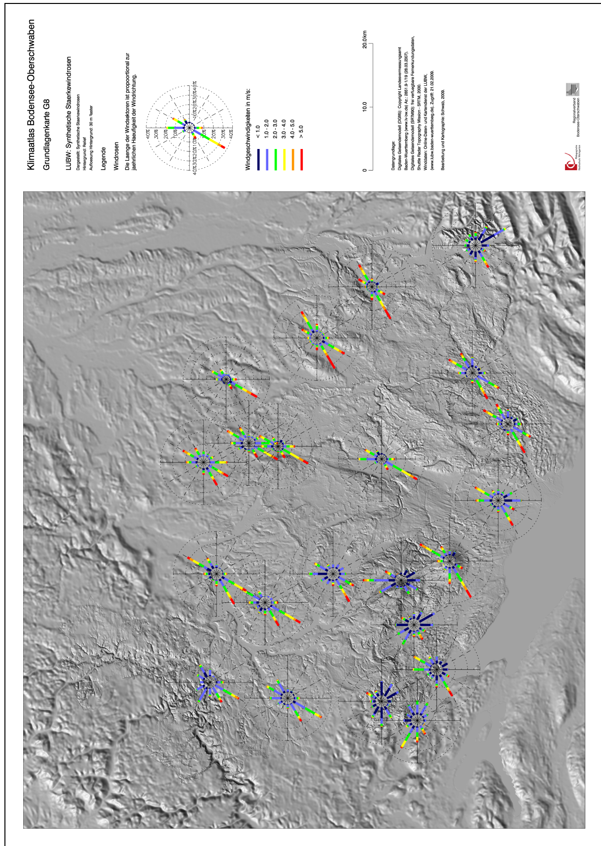
Karte 17: Synthetische Stärkewindrosen der LUBW im Untersuchungsraum (LUBW, 2009). (=Karte G8 im eigentlichen Kartenteil der Klimaanalyse).
