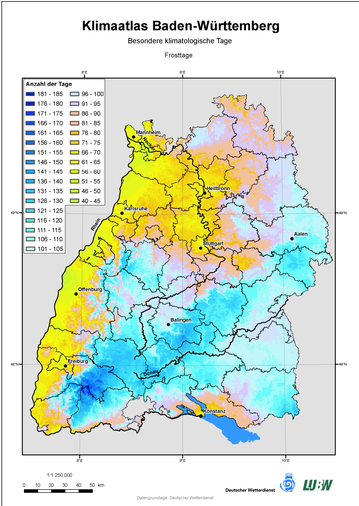
Karte 6: Anzahl der Frosttage in Baden-Württemberg (LUBW, 2006).
