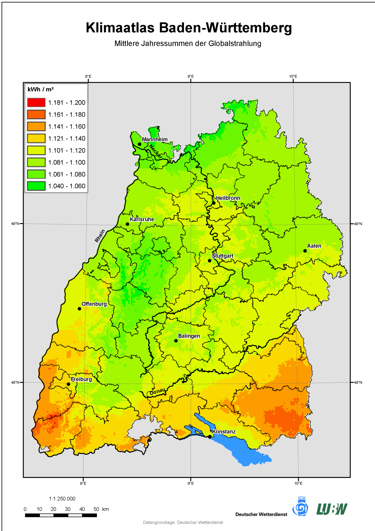
Karte 10: Mittlere Jahressummen der Globalstrahlung in Baden-Württemberg (LUBW, 2006).
