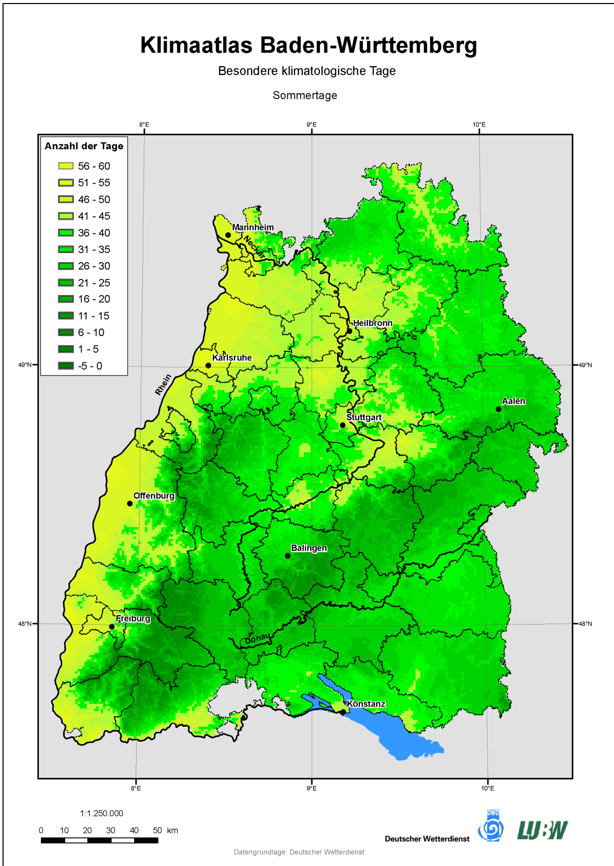
Karte 5: Anzahl der Sommertage in Baden-Württemberg (LUBW, 2006).
