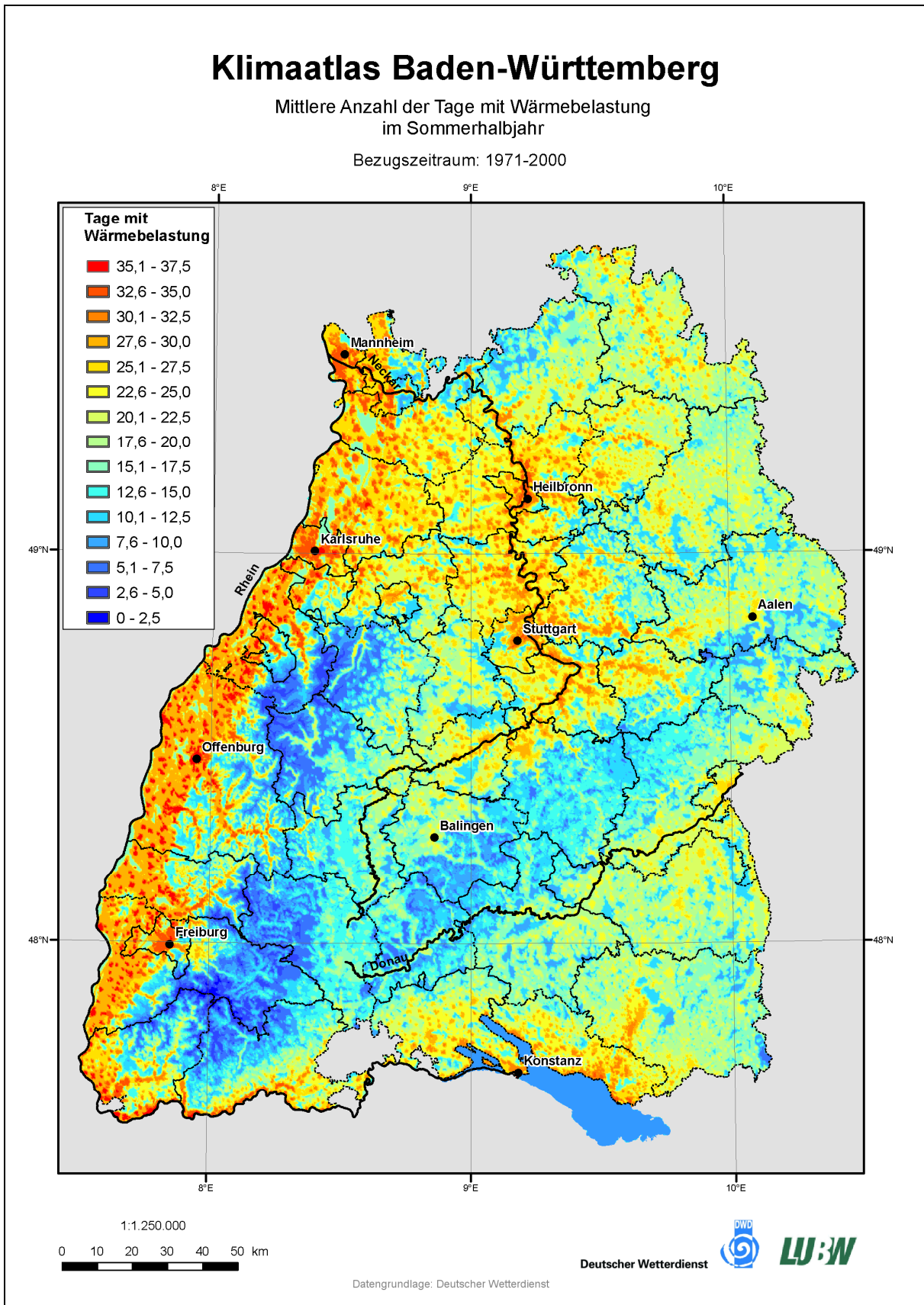
Karte 21: Mittlere Anzahl der Tage mit Wärmebelastung im Sommerhalbjahr (LUBW, 2006).
