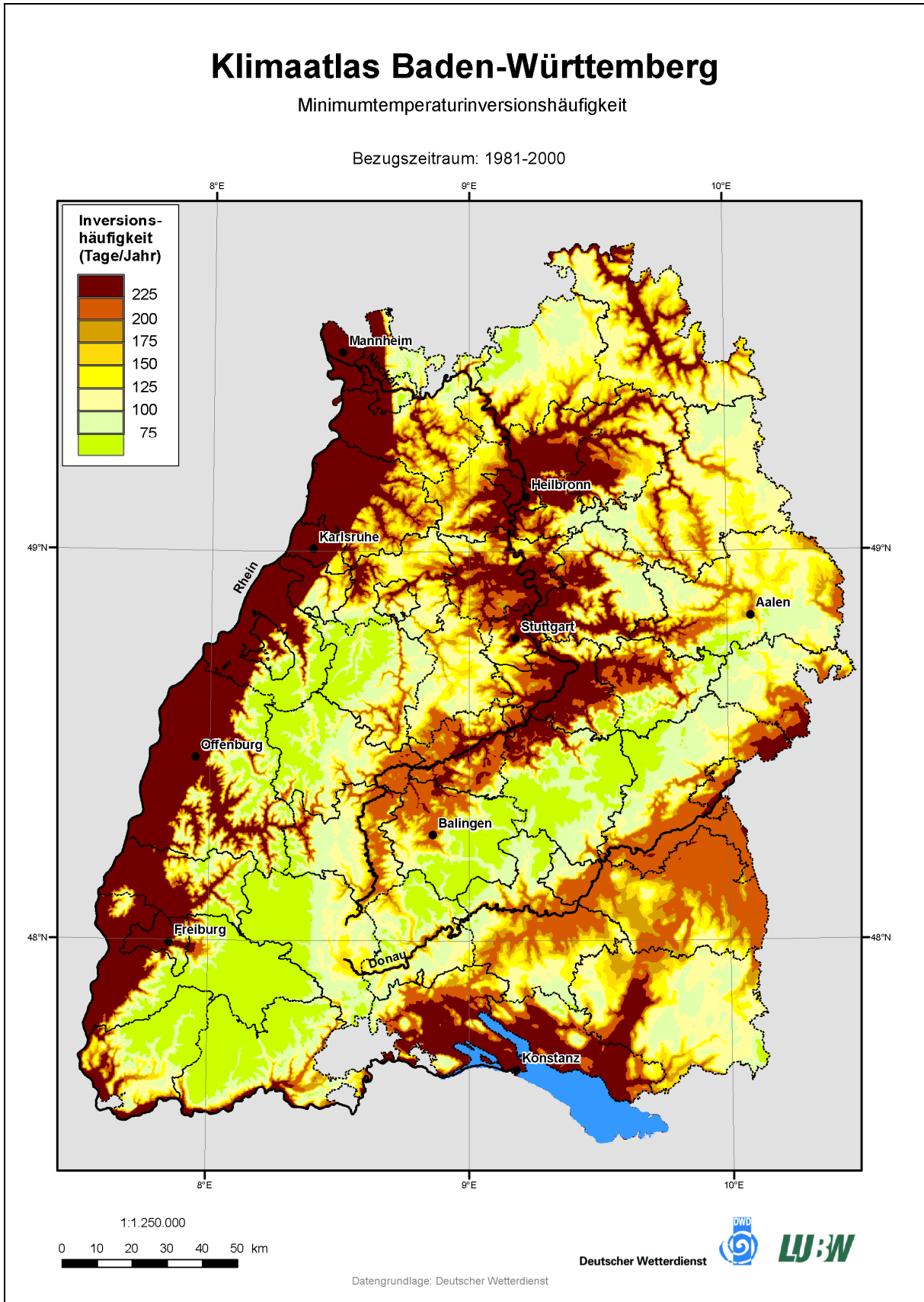
Karte 18: Minimumtemperaturinversionshäufigkeit (LUBW, 2006).
