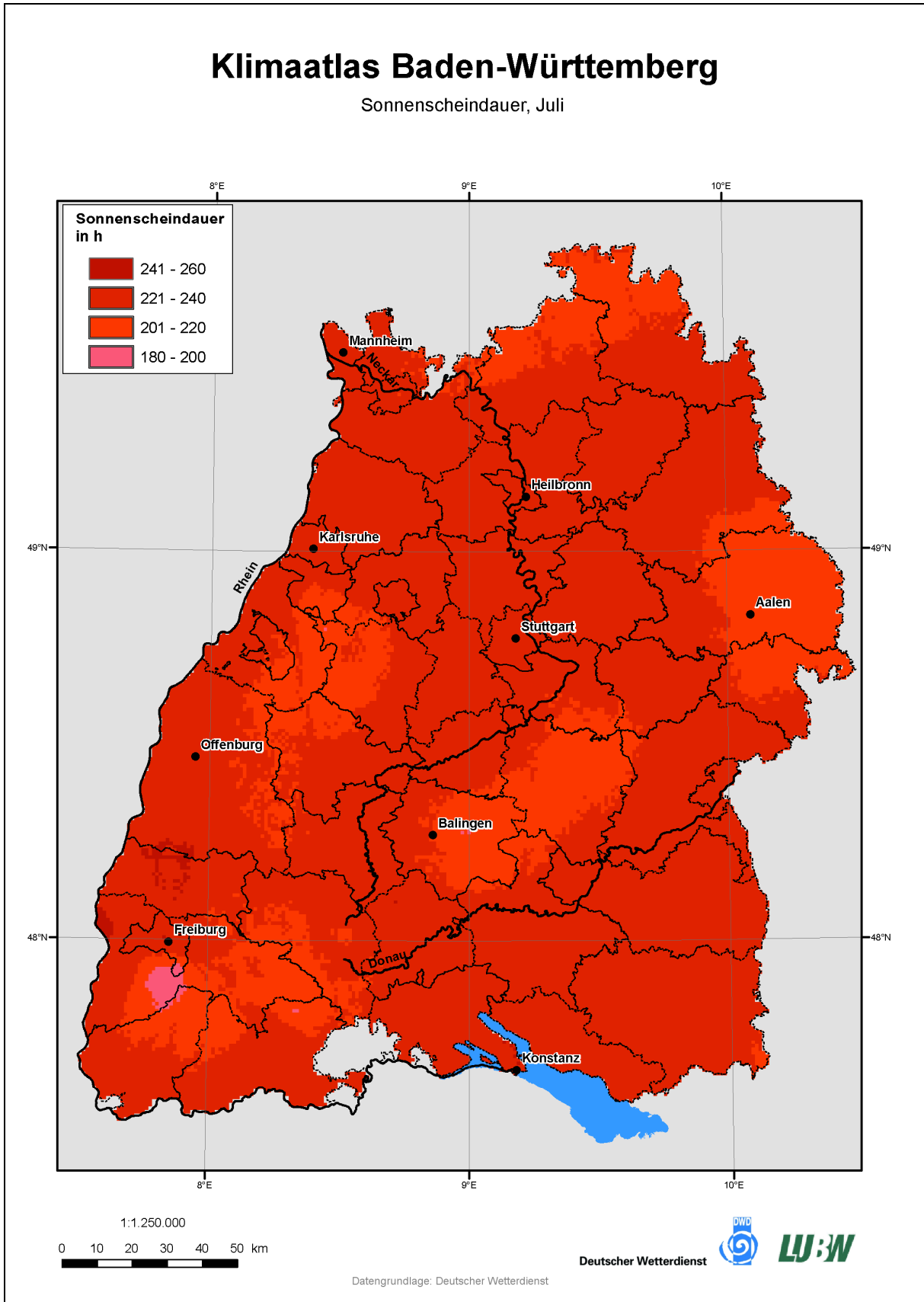
Karte 8: Sonnenscheindauer im Juli in Baden-Württemberg (LUBW, 2006).
