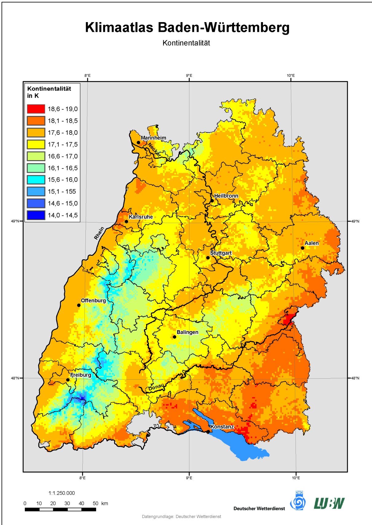
Karte 1: Kontinentalität als Jahresschwankung der Lufttemperatur in Baden-Württemberg (LUBW, 2006).
