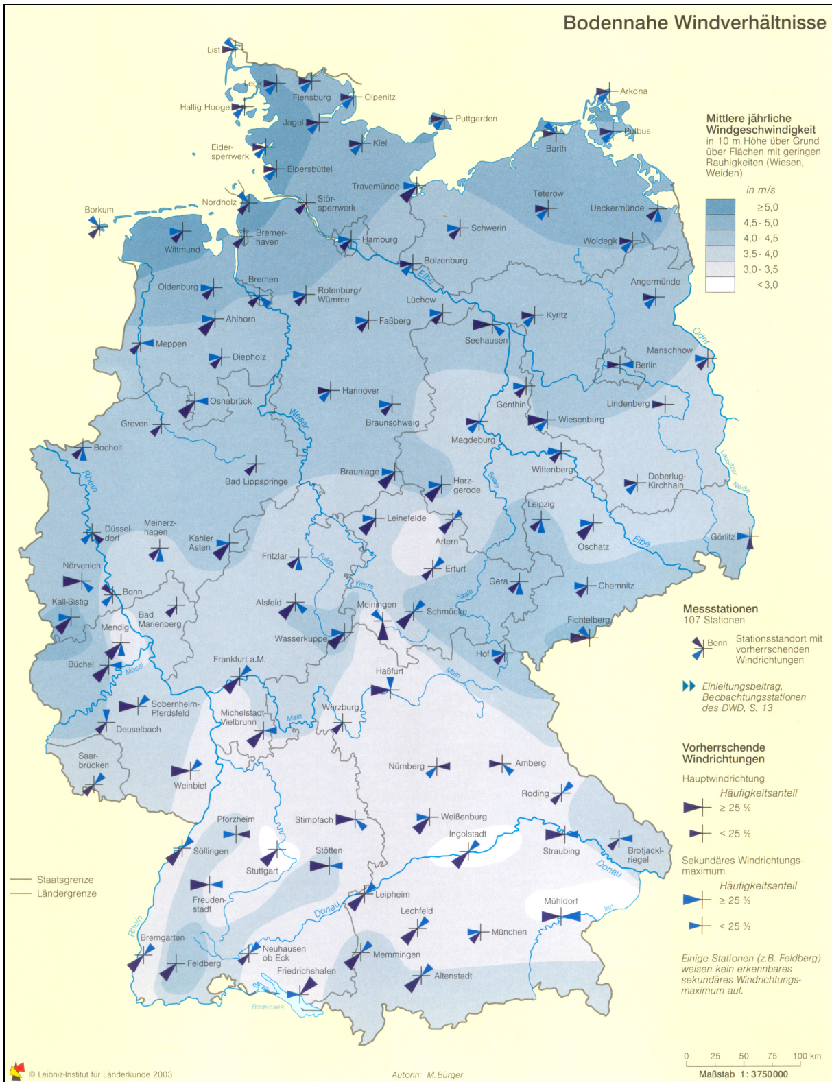
Karte 14: Bodennahe Windverhältnisse in Deutschland (aus: Nationalatlas, 2003).
