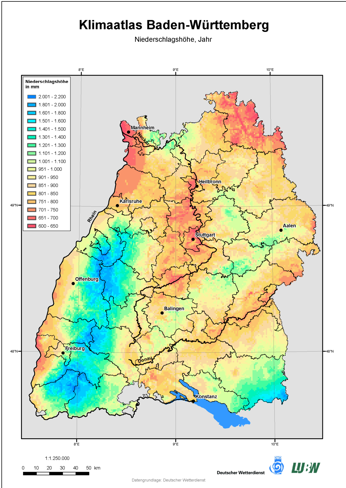
Karte 11: Jährliche Niederschlagshöhe in Baden-Württemberg (LUBW, 2006).
