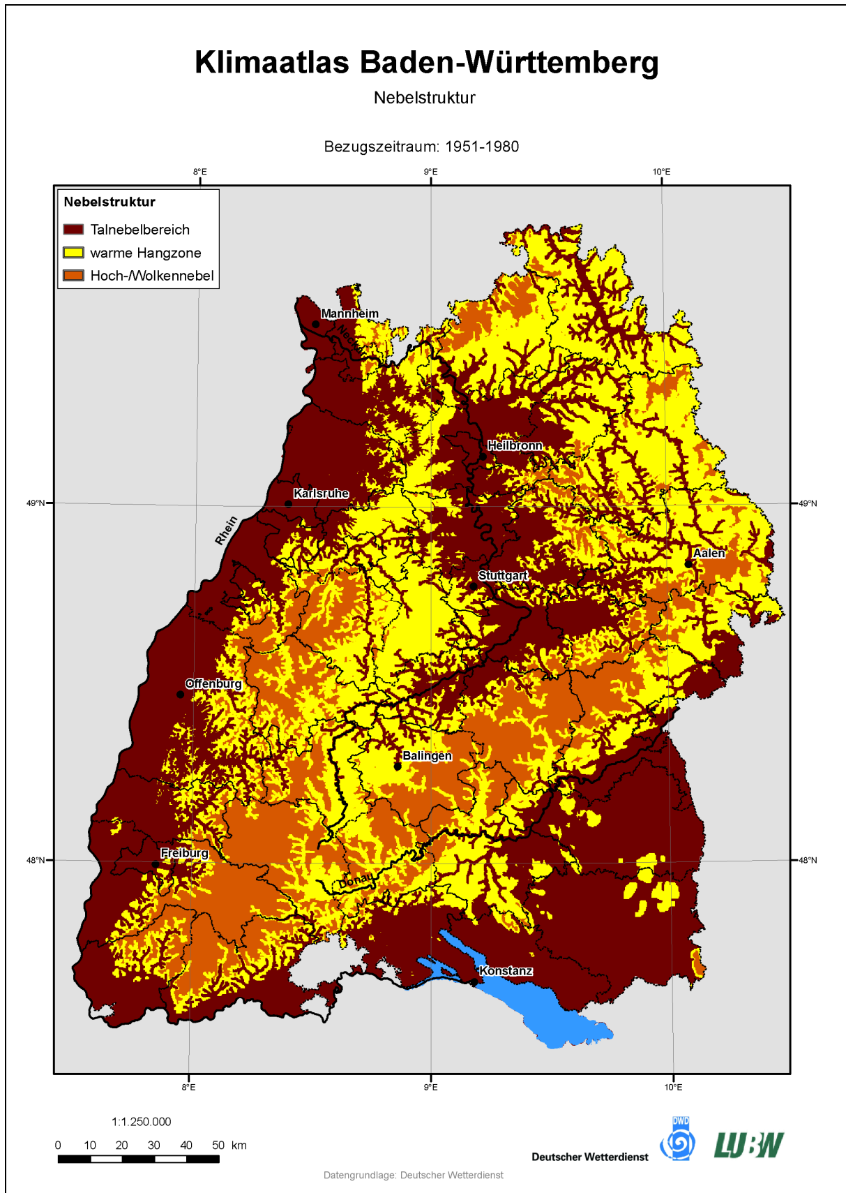
Karte 12: Nebelstruktur in Baden-Württemberg (LUBW, 2006).
