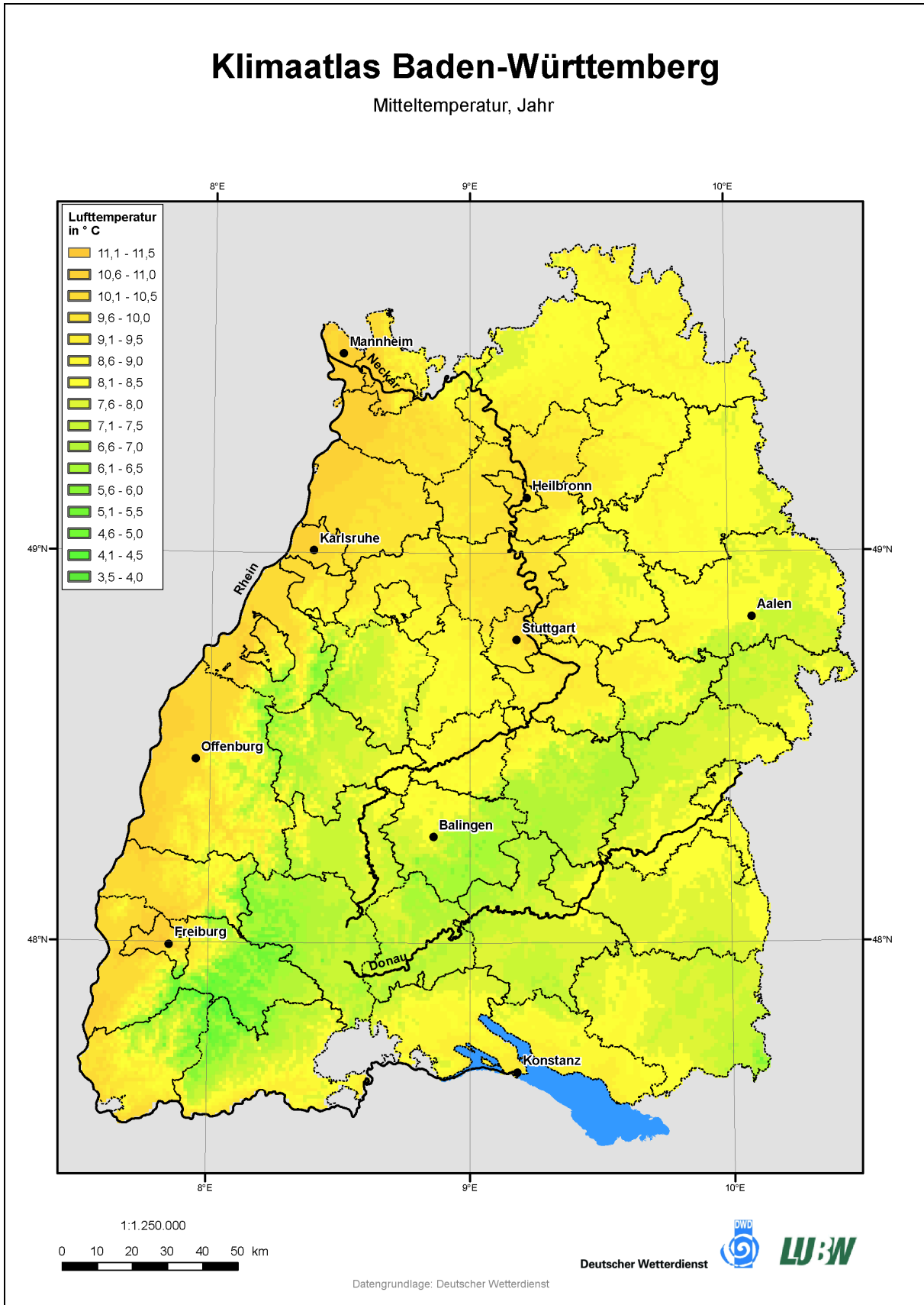
Karte 4: Jahresmittelwerte der Lufttemperatur in Baden-Württemberg (LUBW, 2006).
