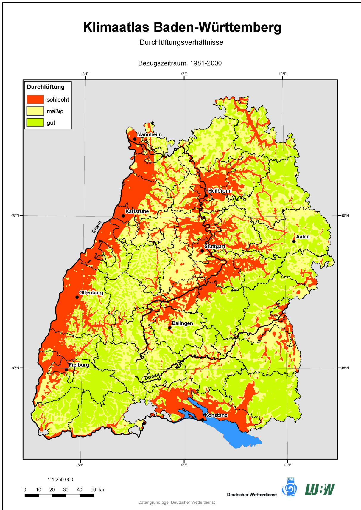
Karte 19: Durchlüftungsverhältnisse (LUBW, 2006).
