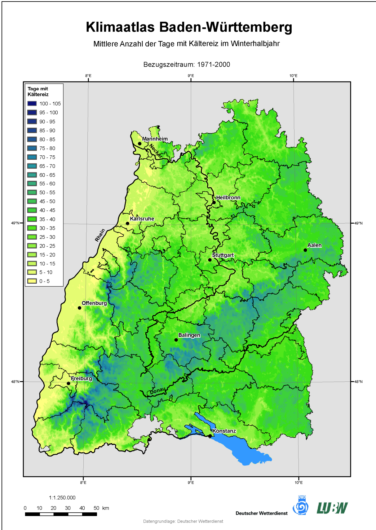
Karte 20: Mittlere Anzahl der Tage mit Kältereiz im Winterhalbjahr (LUBW, 2006).
