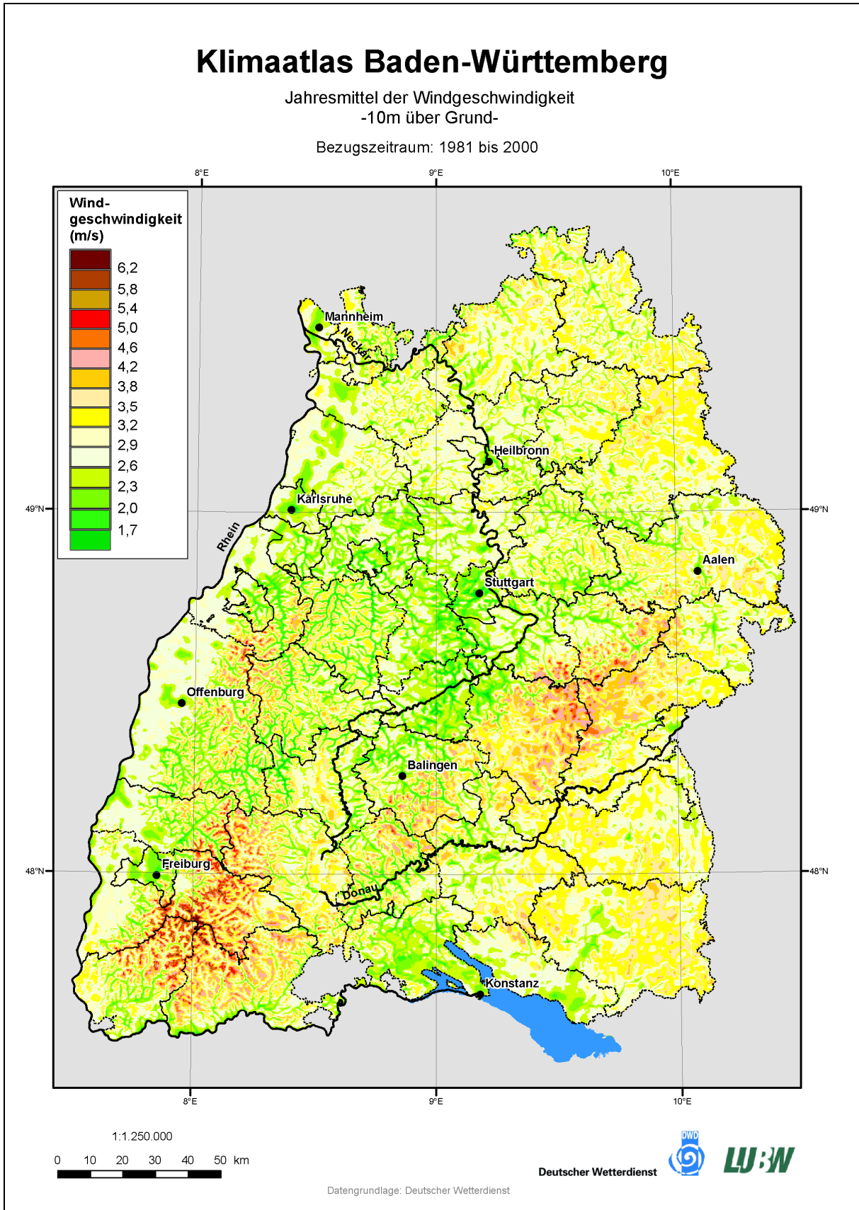
Karte 15: Jahresmittel der Windgeschwindigkeit in Baden-Württemberg (LUBW, 2006).
