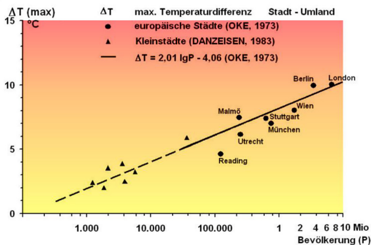
Abbildung 4: Maximale Temperaturunterschiede für europäische Städte unterschiedlicher Größe (aus: Städtebauliche Klimafibel, Online-Version, 2009).
