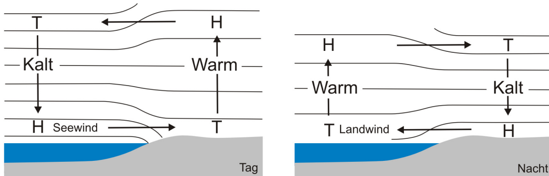
Abbildung 7: Seewind am Tag und Landwind in der Nacht als Ergebnis der unterschiedlichen Erwärmung von Land- und Wasseroberflächen und der daraus resultierenden Druckfelder. Die Linien stellen isobare Flächen dar. (Entwurf: Schwab, verändert nach Gossmann, S. 139)
