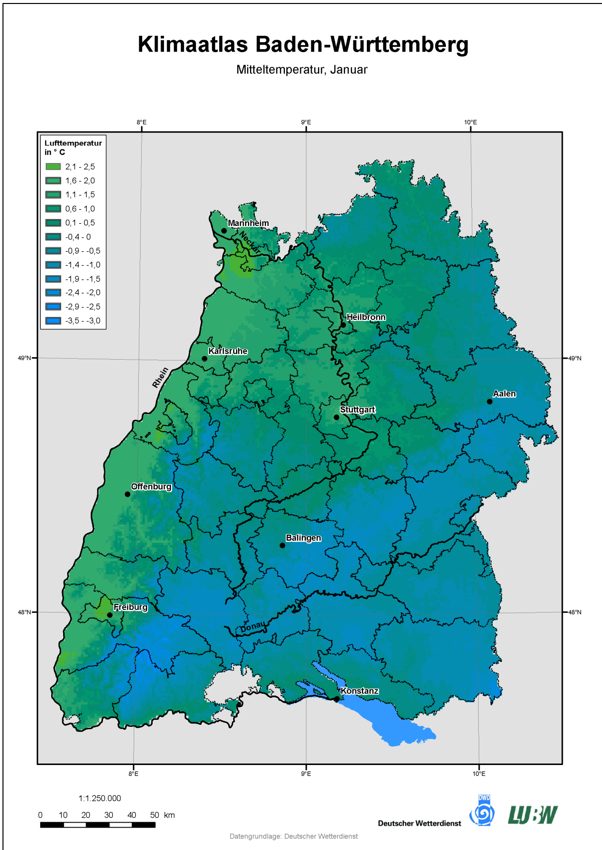
Karte 2: Mittelwert der Lufttemperaturen im Januar in Baden-Württemberg (LUBW, 2006).
