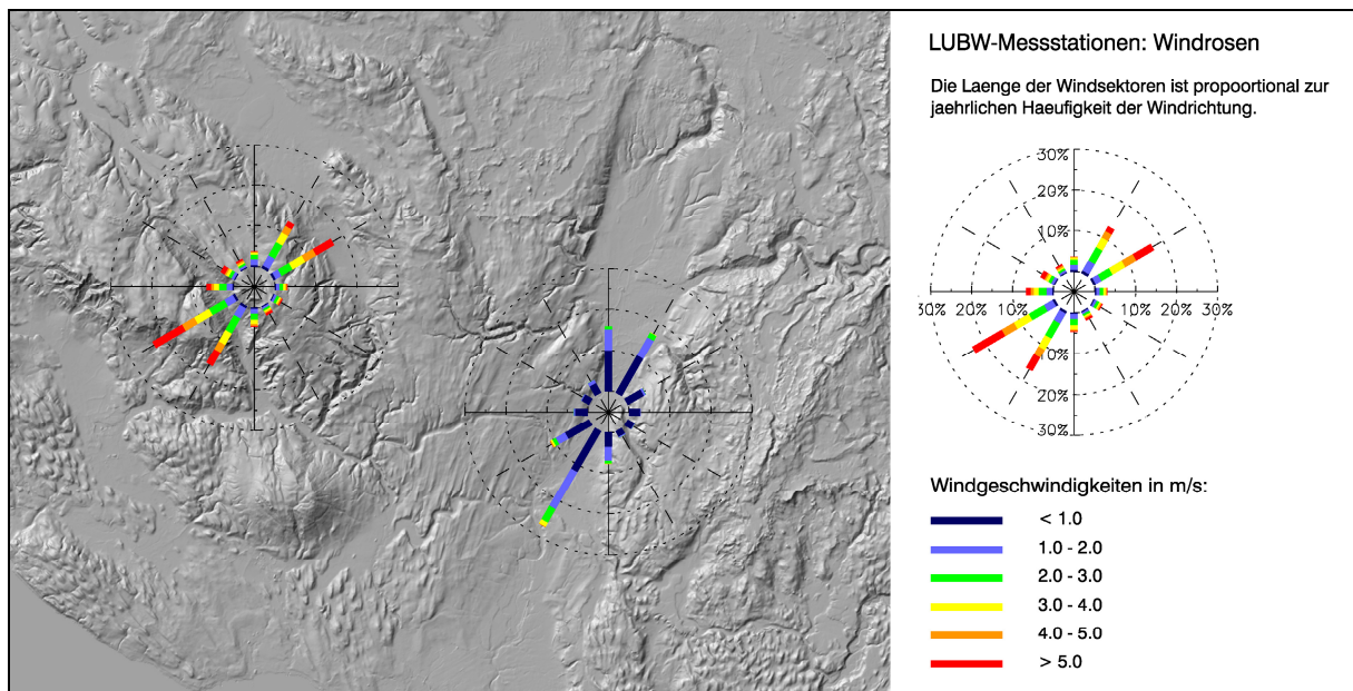
Abbildung 27: Stärkewindrosen der LUBW-Messstationen Illmensee und Ravensburg. (Ausschnitt aus Anhang, Karte 16).
