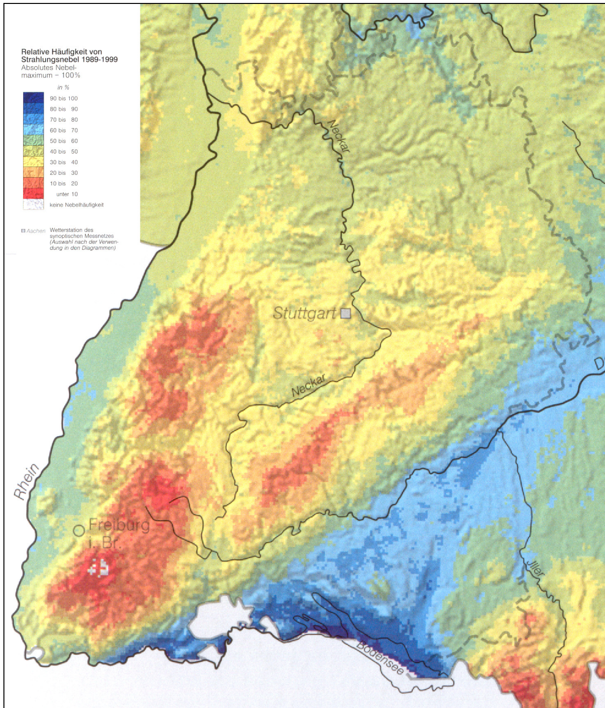
Karte 13: Relative Häufigkeit von Strahlungsnebel (Ausschnitt aus: Nationalatlas, 2003).
