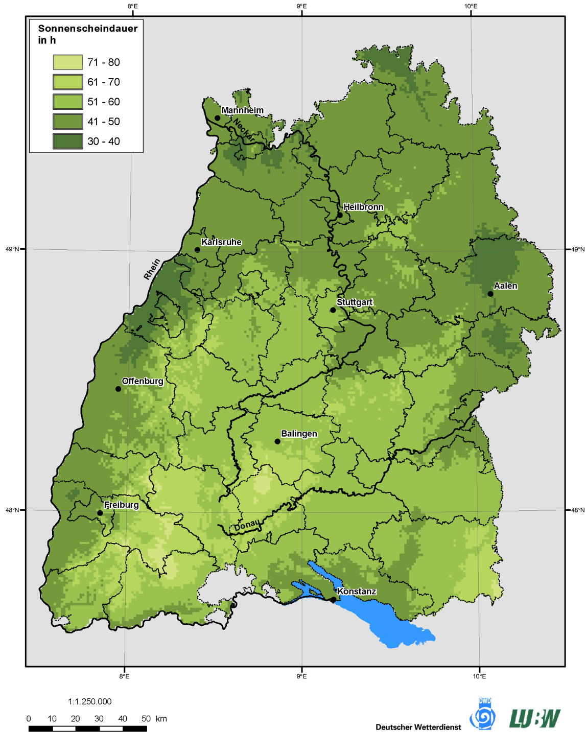
Karte 7: Sonnenscheindauer im Januar in Baden-Württemberg (LUBW, 2006).
