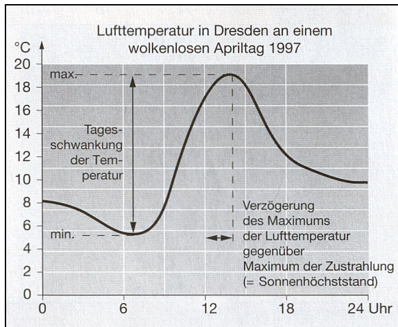
Abbildung 2: Typischer Tagesgang der Lufttemperatur an einem wolkenlosen Apriltag in Dresden 1997. (aus: BAUER et al, S. 82)
